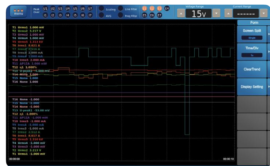
Trend Display
